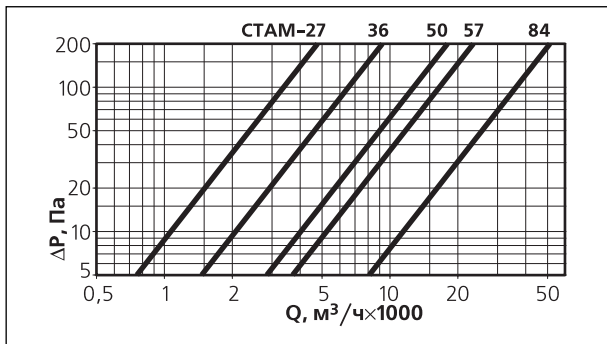
Компоновка 010, 011
